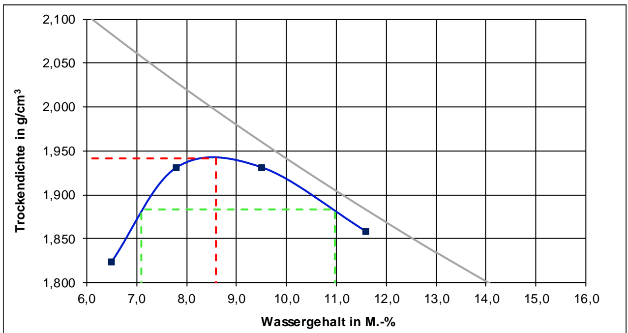
Proctorkurve des untersuchten RC-Materials 0/45
