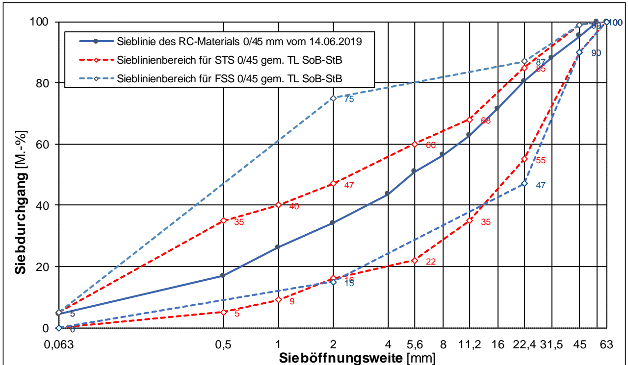
Korngrößenverteilung des untersuchten RC-Materials 0/45 mit Sieblinienbereich für Schottertrag- und Frostschuttschichten 0/45 mm gemäß TL SoB-StB /7/
