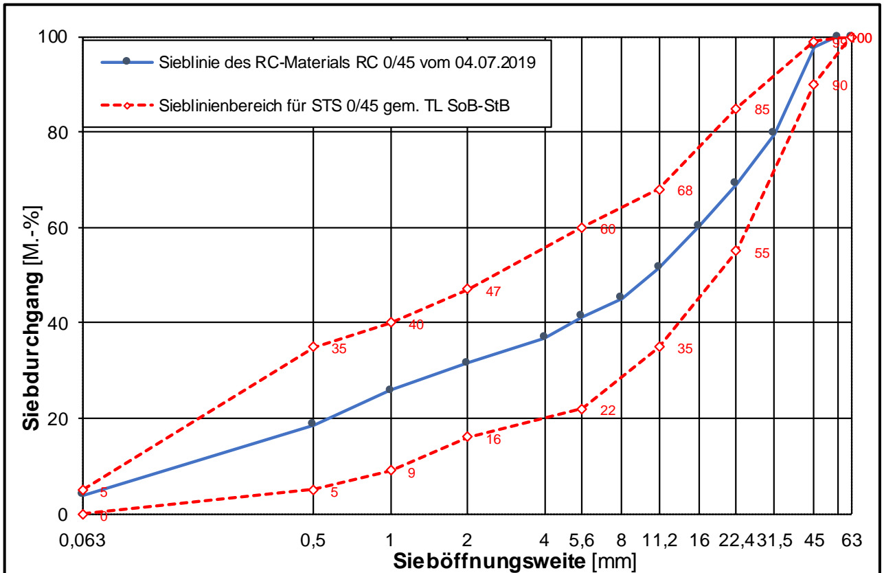
Korngrößenverteilung des untersuchten RC-Materials 0/45 mit Sieblinienbereich für Schottertrag-schicht 0/45 mm gemäß TL SoB-StB /7/
