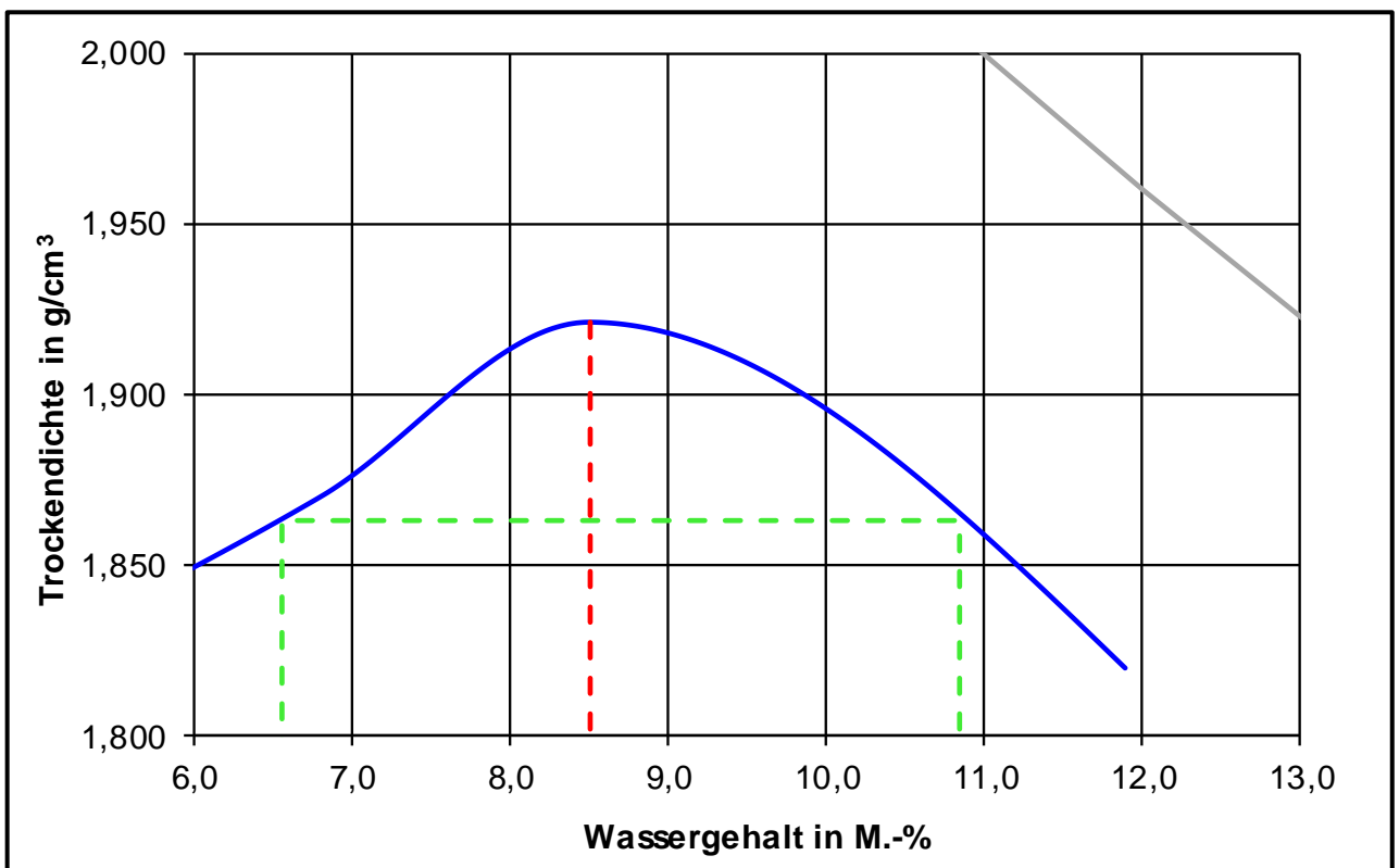
Proctorkurve des untersuchten RC-Materials 0/45
