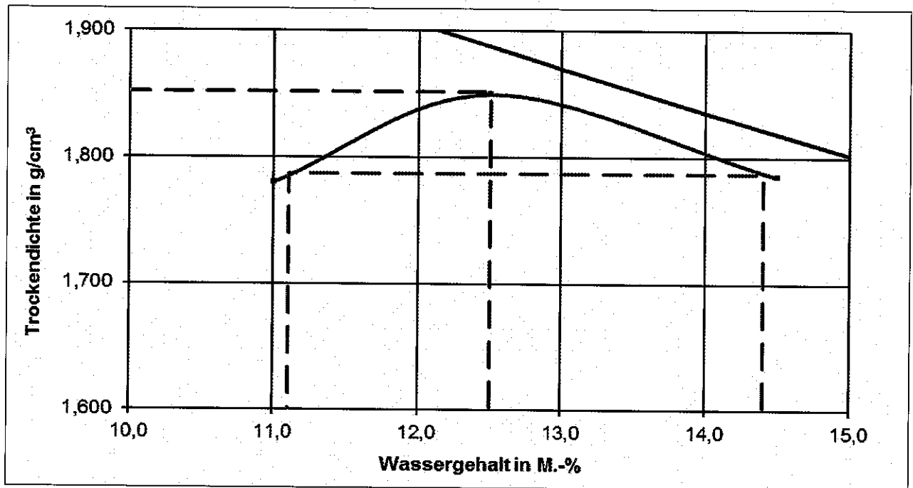
Proctorkurve des untersuchten RC-Materials 0/45 (aus Prüfbericht F 17/02/0177 – I/2017)
