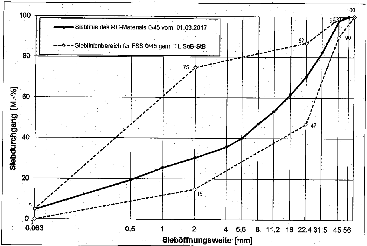
Korngrößenverteilung des untersuchten RC-Materials 0/45 mit Sieblinienbereich für Frostschuttschichten 0/45 mm gemäß TL SoB-StB /8/
